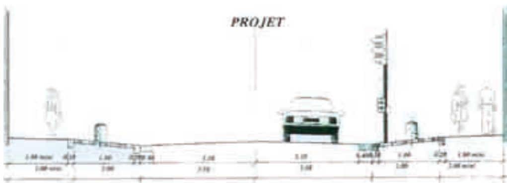
PROFIL SECTION COURANTE TYPE.
