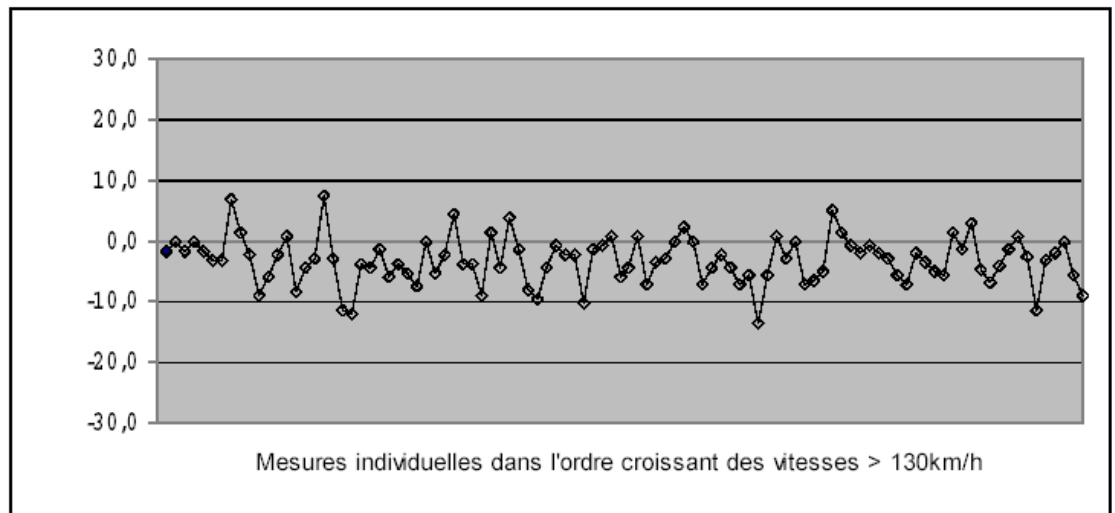
Figure 16 : Dispersion en % des écarts en fonction des vitesses croissantes V>130 sans correction
