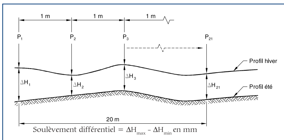
Figure 3-6 Soulèvements différentiels
