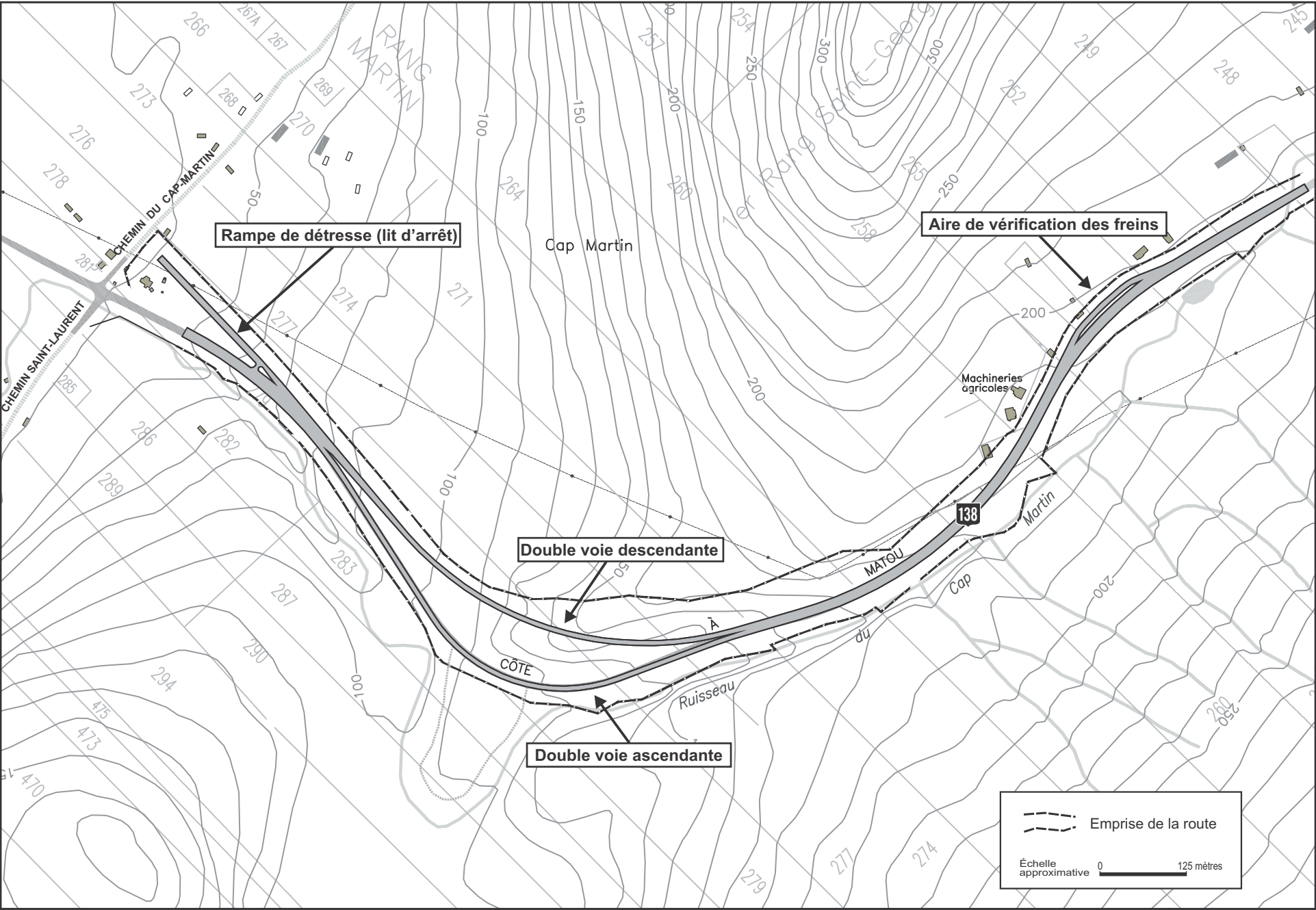
Figure 1: Aménagement de la route 138, dans le secteur de la côte à Matou à Saint-Urbain
